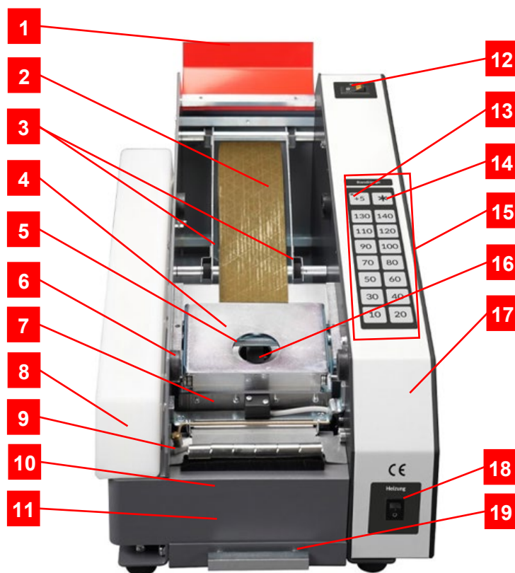
Abbildung 1: Aufbau und Komponenten des Gerätes
